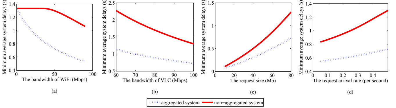
Fig. 9. Minimum average system delays in terms of (a) B_1 ; (b) B_2 ; (c) \mu ; (d) \lambda
